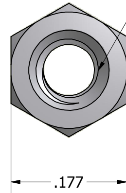
M2.5 x 0.45-6H Thru
