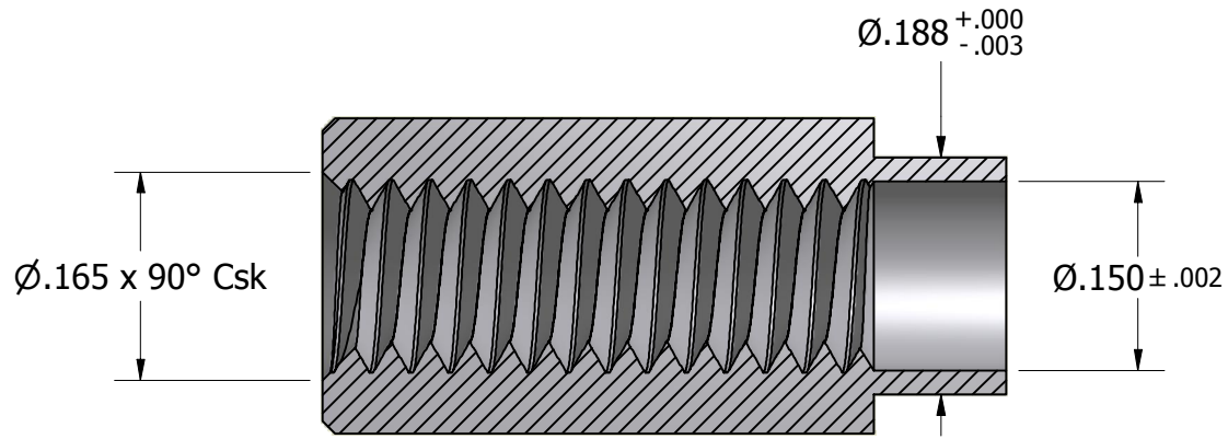
SECTION A-A
