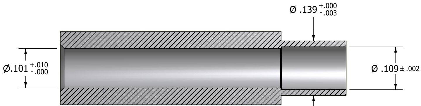
SECTION A-A
