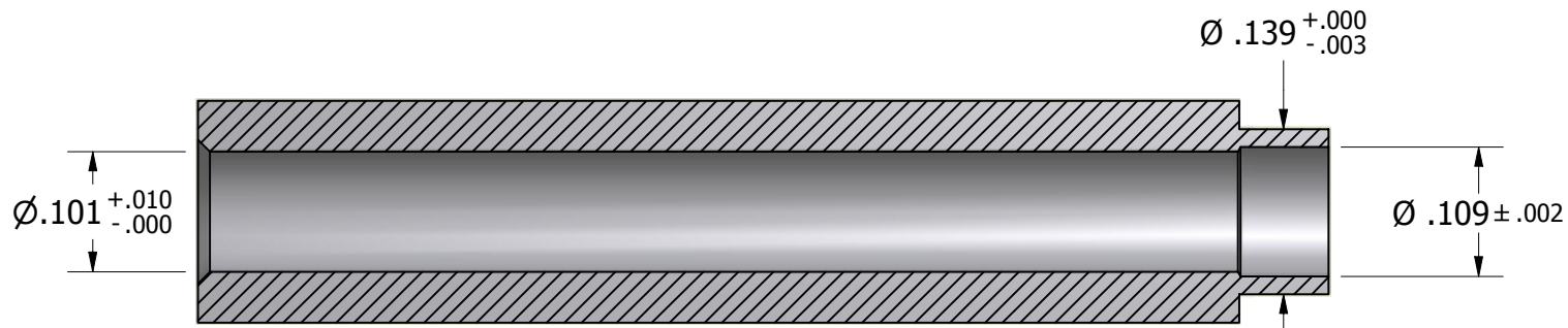
SECTION A-A
