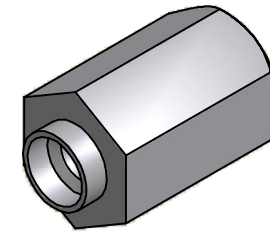
ISO SCALE 2 : 1
