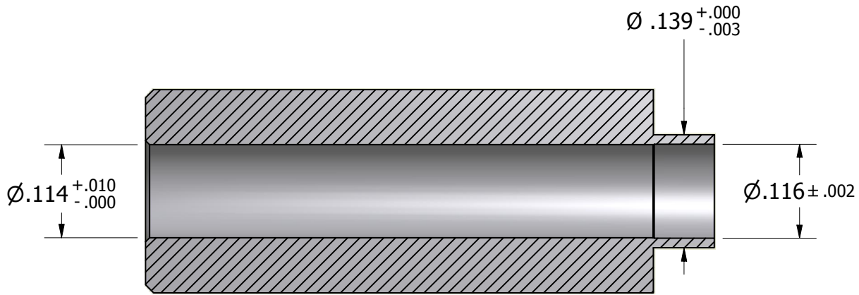
SECTION A-A
