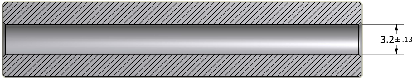
SECTION A-A
