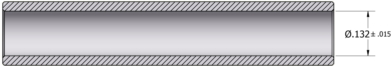
SECTION A-A
