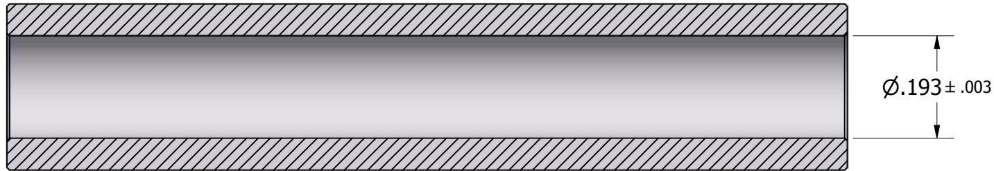
SECTION A-A
