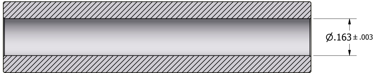
SECTION A-A
