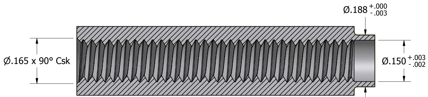
SECTION A-A
