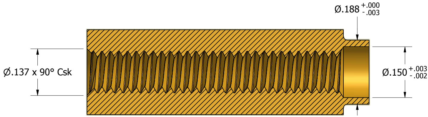
SECTION A-A
