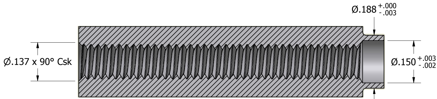
SECTION A-A
