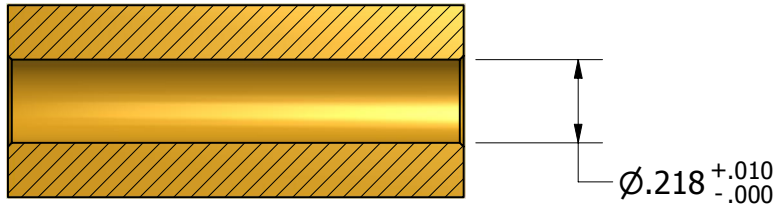
SECTION A-A
