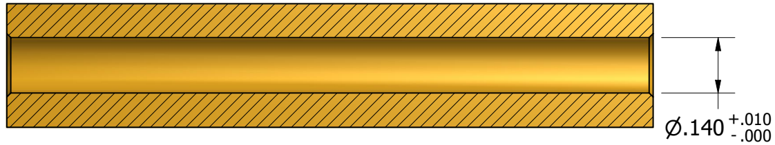
SECTION A-A
