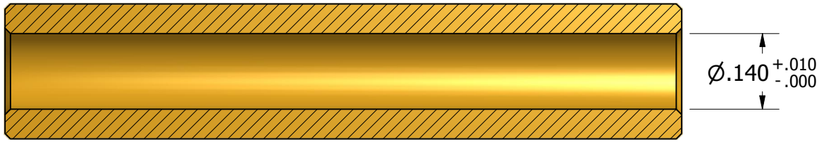
SECTION A-A
