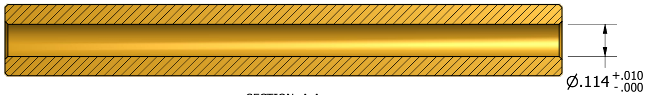
SECTION A-A
