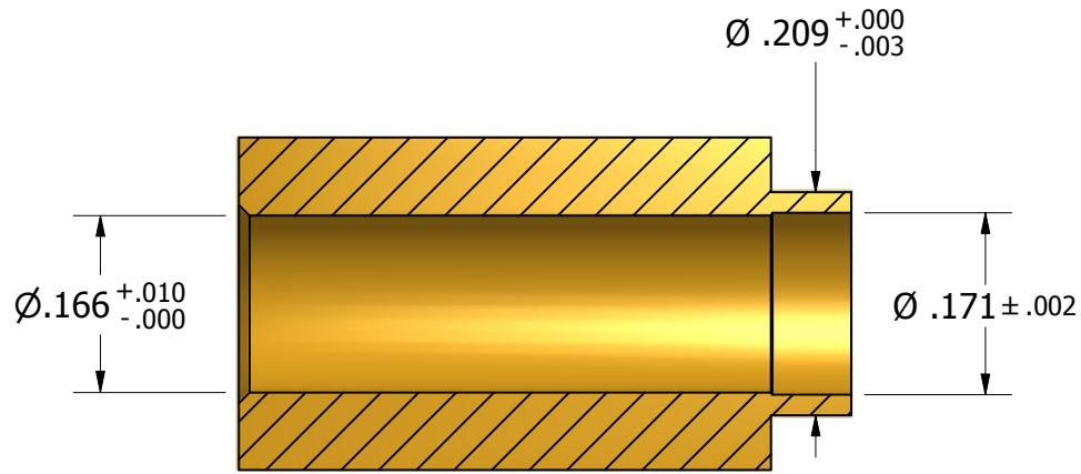
SECTION A-A
