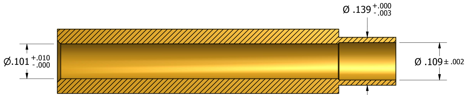
SECTION A-A
