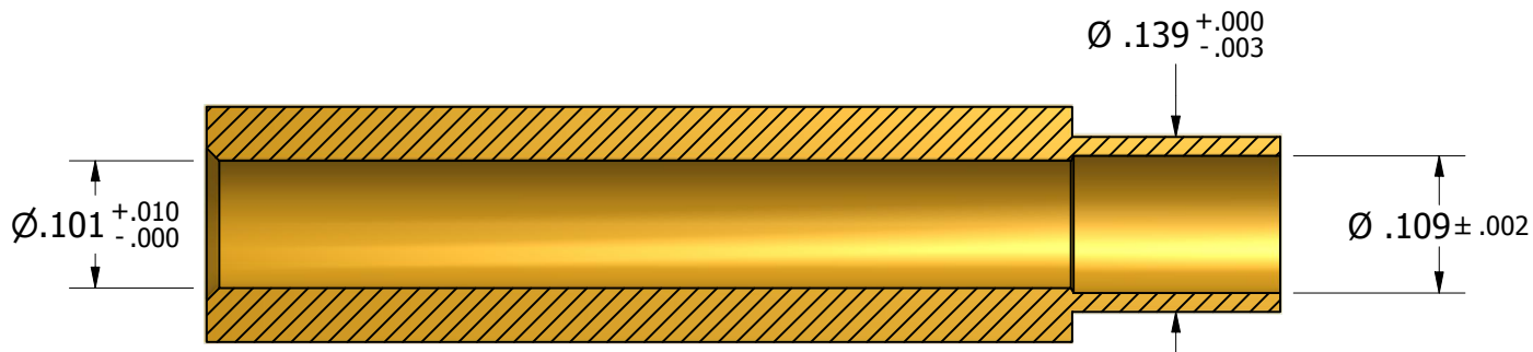
SECTION A-A
