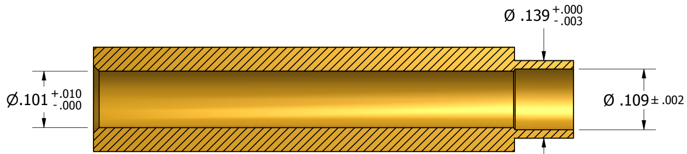
SECTION A-A
