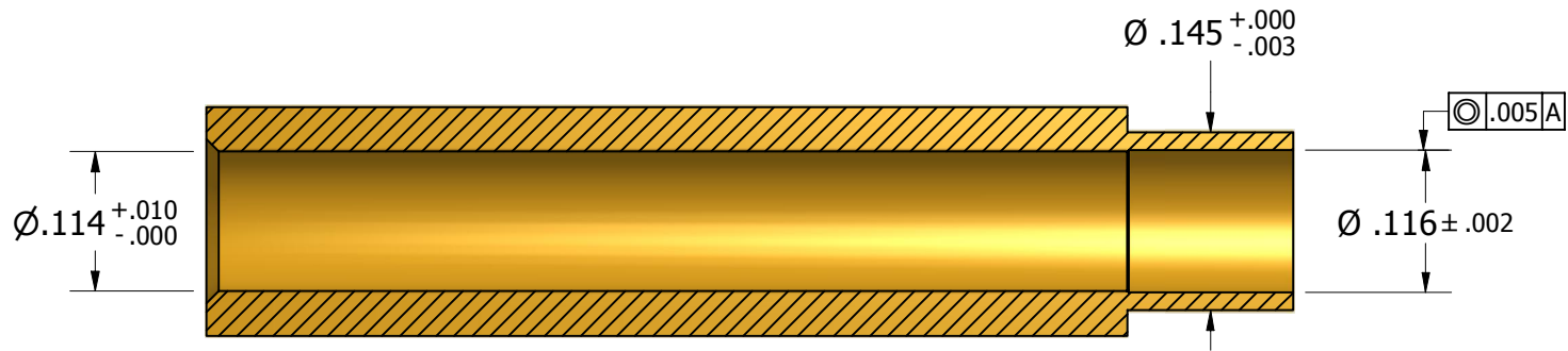
SECTION A-A
