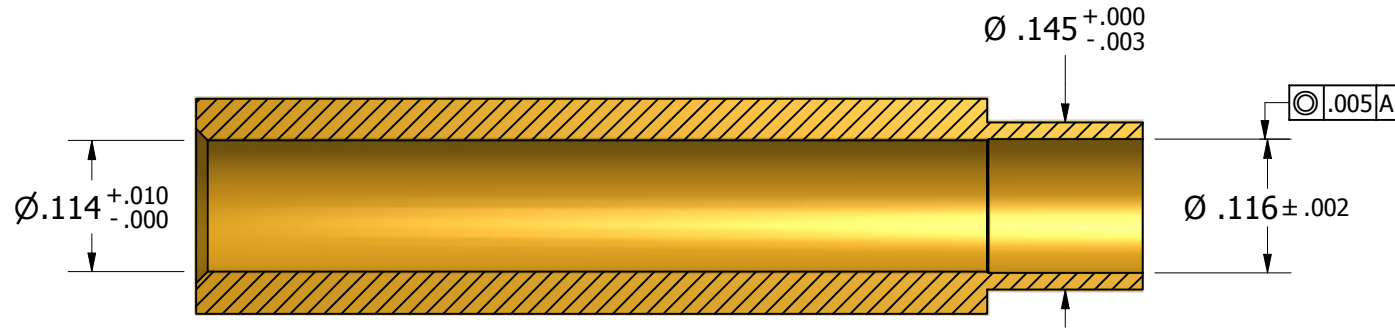
SECTION A-A
