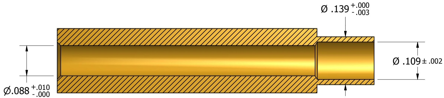
SECTION A-A
