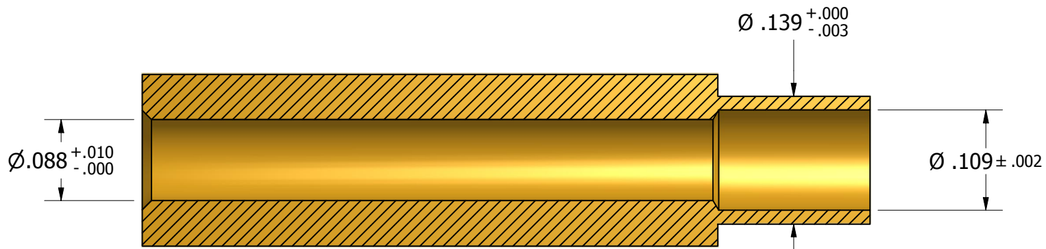
SECTION A-A
