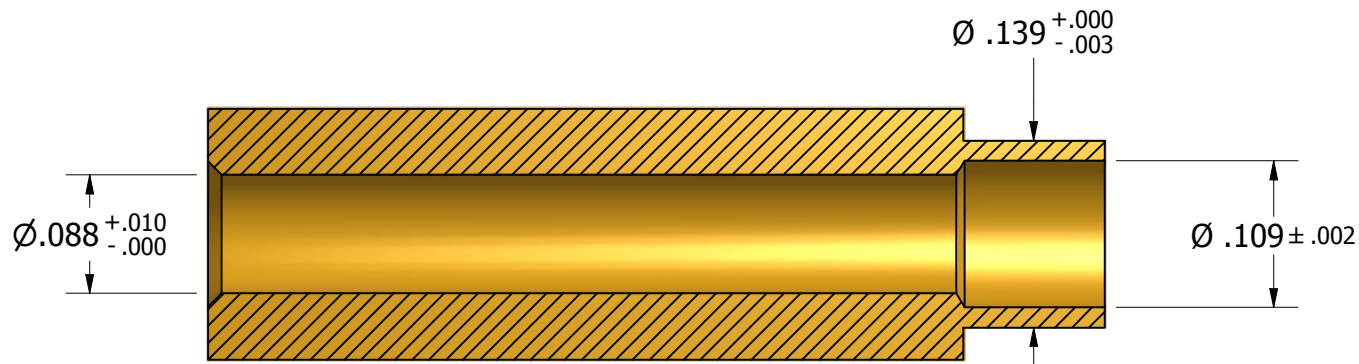
SECTION A-A
