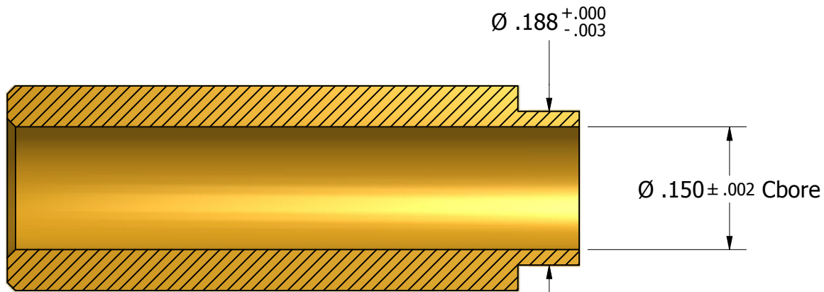
SECTION A-A
