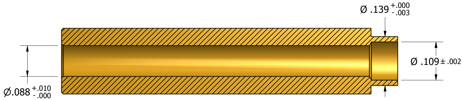
SECTION A-A
