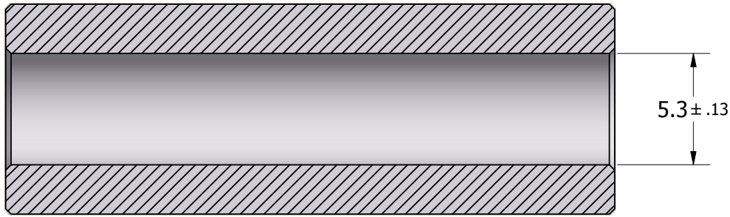
SECTION A-A
