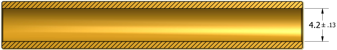
SECTION A-A
