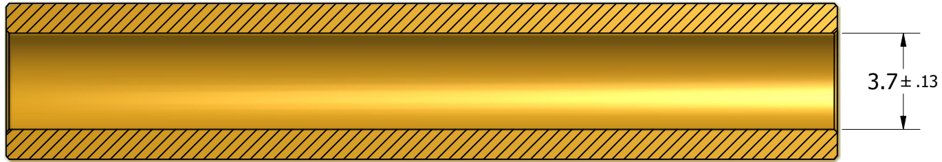
SECTION A-A
