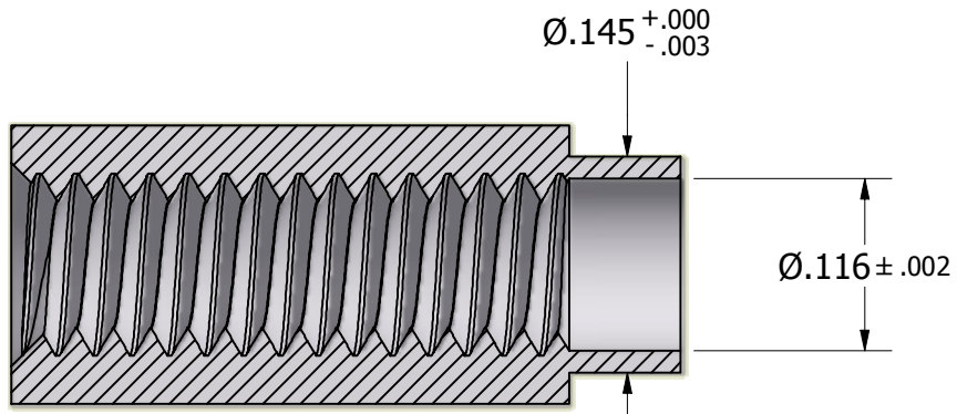
SECTION A-A
