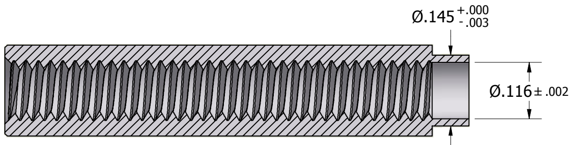
SECTION A-A
