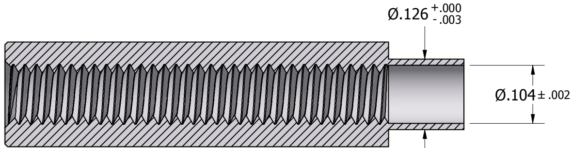
SECTION A-A
