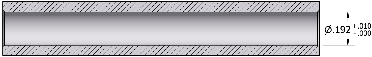
SECTION A-A
