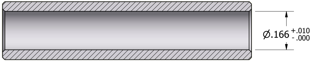
SECTION A-A
