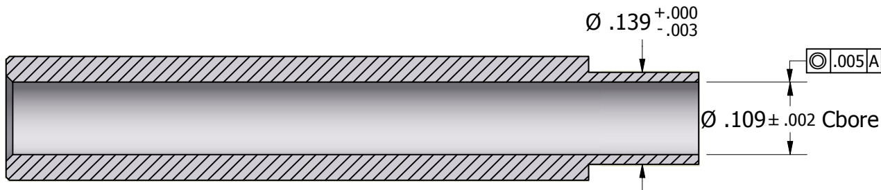
SECTION A-A
