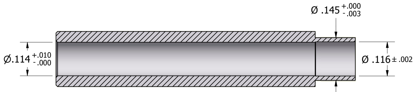
SECTION A-A
