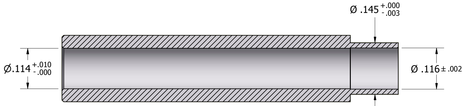
SECTION A-A
