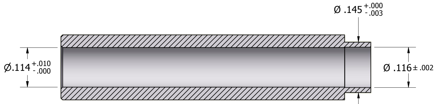
SECTION A-A
