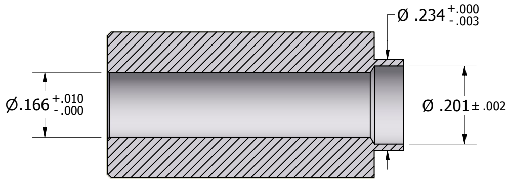
SECTION A-A
