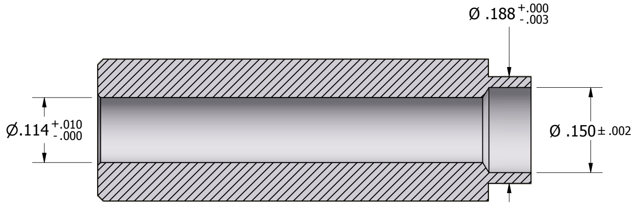
SECTION A-A
