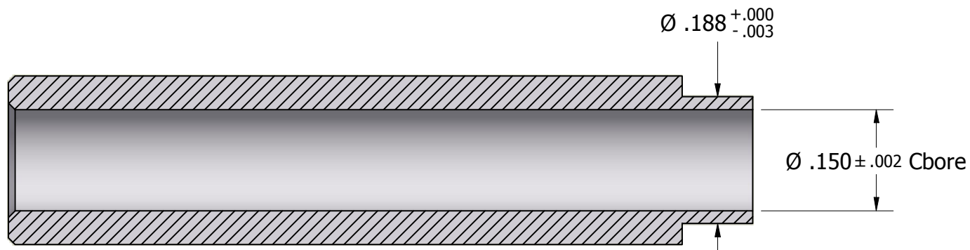
SECTION A-A
