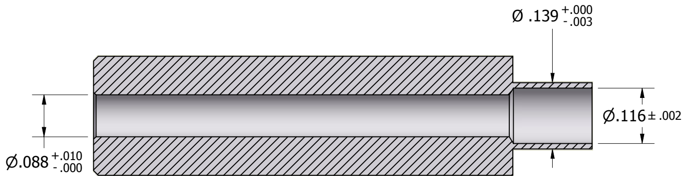
SECTION A-A
