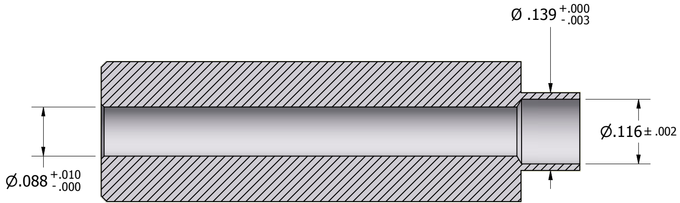
SECTION A-A
