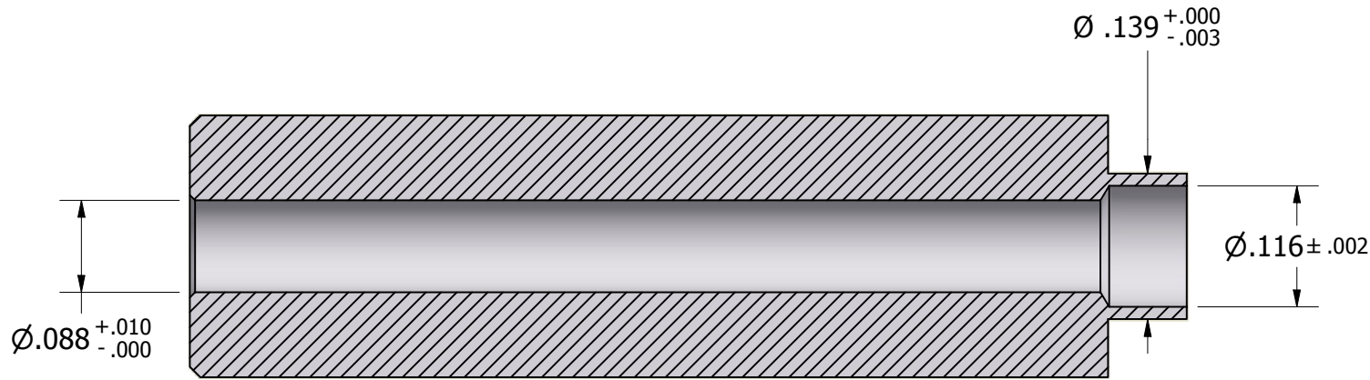
SECTION A-A
