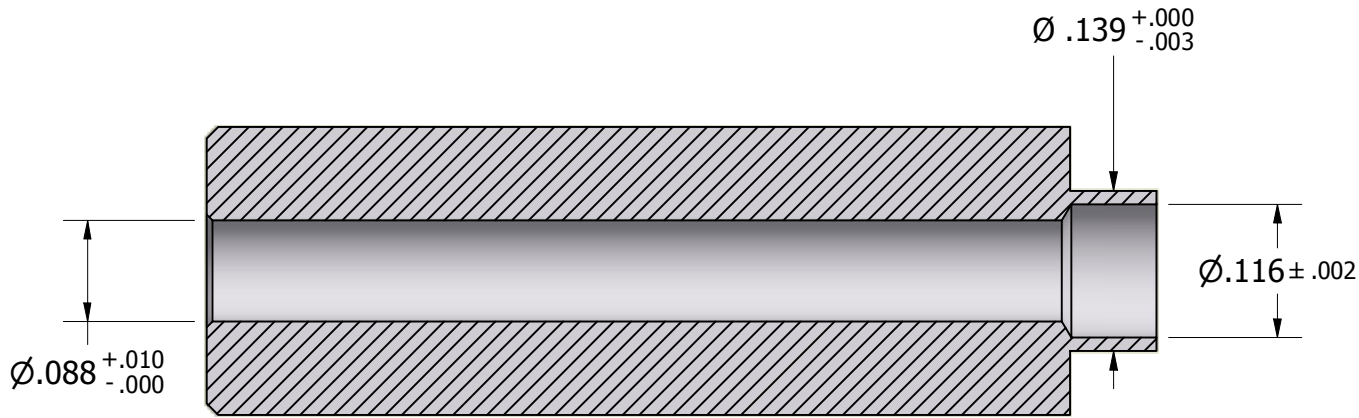
SECTION A-A
