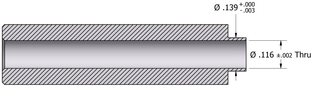
SECTION A-A
